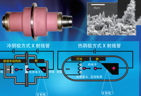
冷阴极X射线管
