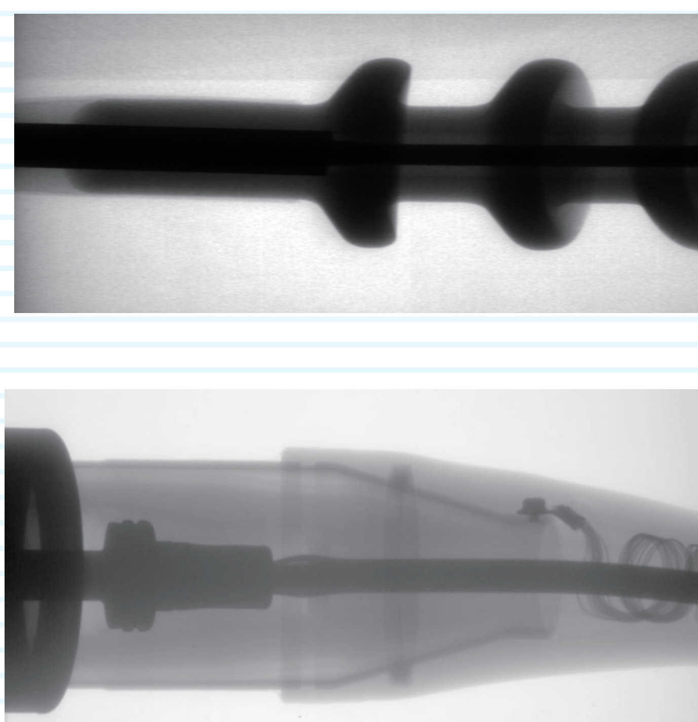
电线端头检测
