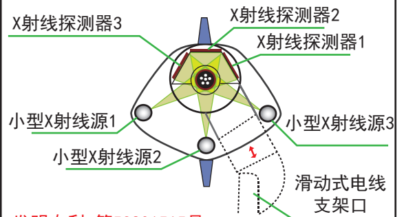
三方向检测原理图
