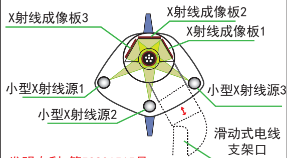
三方向检测原理图
