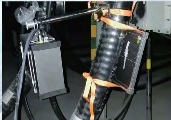
变电站电缆现场检测实例
